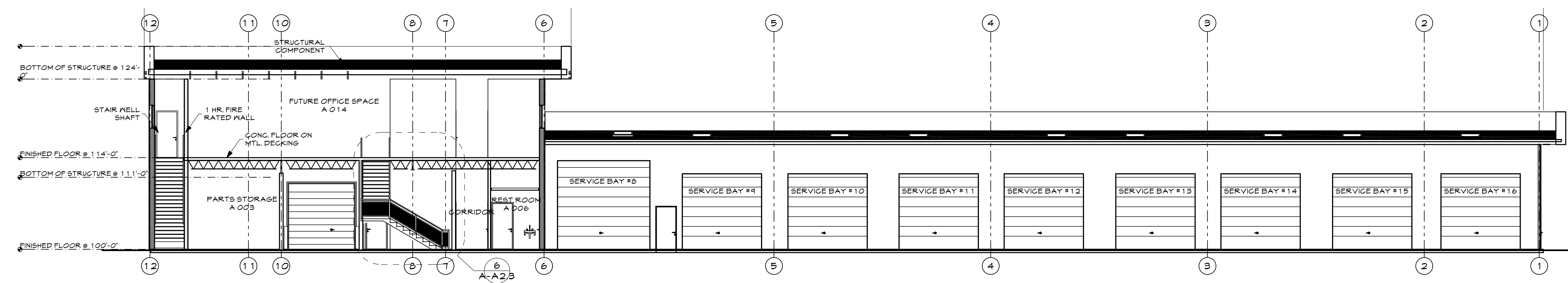
2 SECTION bldg A & B SCALE: 1/8" = 1'-0"
