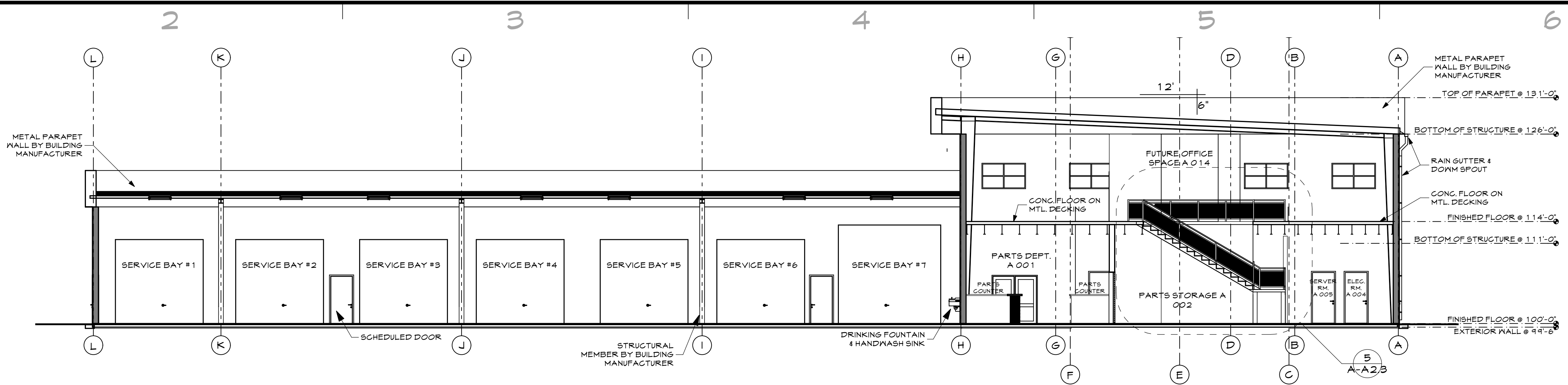
1 SECTION bldg A & C SCALE: 1/8" = 1'-0"
